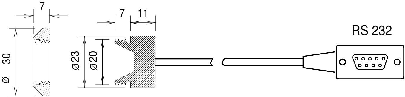
Frontplatte Stärke 1 - 3 mm, Loch Ø 20mm
