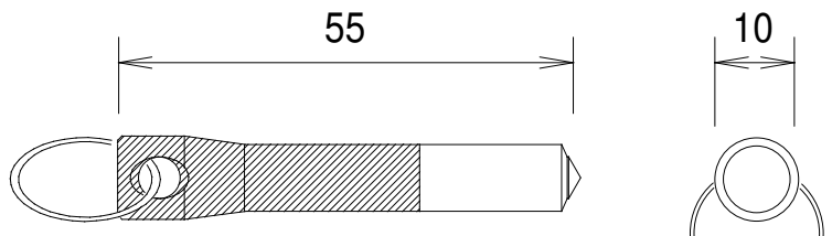
Code-Stift in 10 Farben
